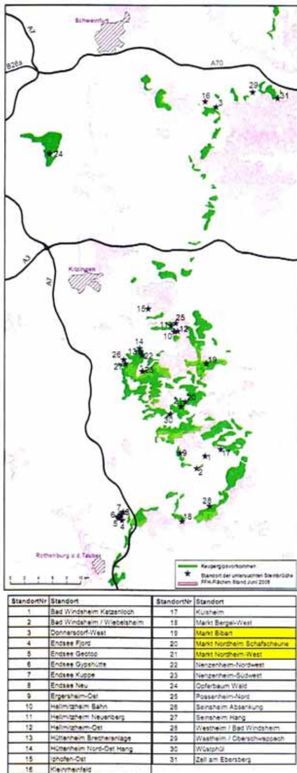
Abb. 1: Keupergipsvorkommen und FFH-Gebiete in Nordbayern.
