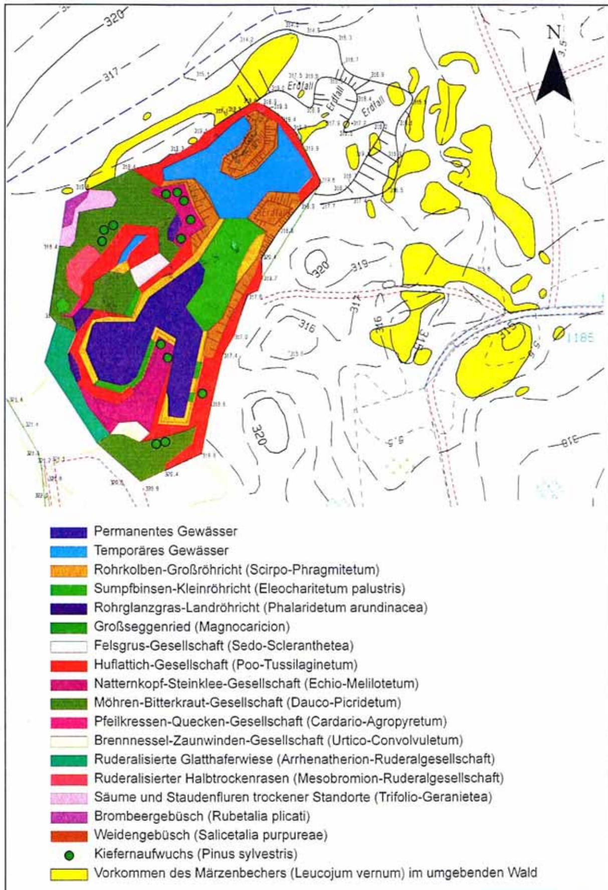
Abb.3: Vegetationskartierung der renaturierten Fläche im ehemaligen Steinbruch bei Markt Bibart.
