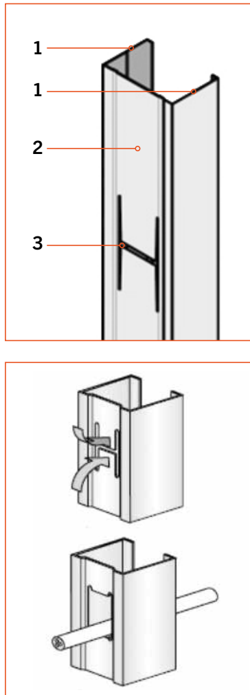
Abb. 14 Beispiel einer Stegöffnung in CW-Profilen 1. Flansch 2. Steg 3. Werkseitige Stanzung (z.B. H-Stanzung)
