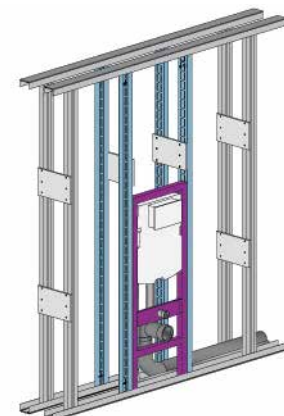
Abb. 11 Beispiel Verlaschung einer Doppelständerwand mit Gipsplattenstreifen
