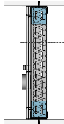
Abb. 9 Beispiel einer kraftschlüssigen Befestigung von UA-Profilen mit Anschlusswinkel am Rohfußboden
