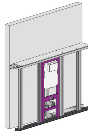
Abb. 10 Beispiel Ausbildung der oberen Abdeckung einer halbhohen Vorsatzschale
