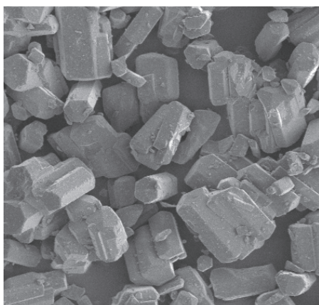
Abb. 4: REM-Aufnahme eines Alpha-Halbhydrats (links) und REM-Aufnahme eines synthetischen Anhydrits
