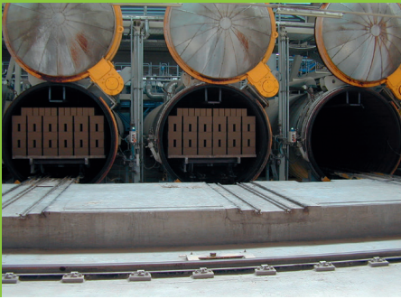
Abb. 7: Autoklaven zur Herstellung von Alpha-Halbhydrat
