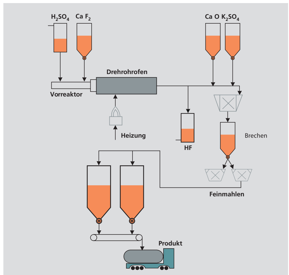
Abb.13: Bestandteile von Synthetischem Anhydrit bei der Herstellung von Flusssäure
