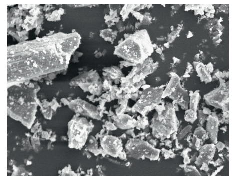
Abb. 9: REM-Aufnahmen von Alpha-Halbhydrat in einem handelsüblichen Fließestrich
