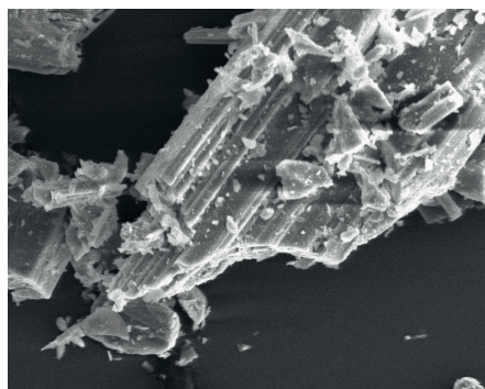
Abb. 9: REM-Aufnahmen von Alpha-Halbhydrat in einem handelsüblichen Fließestrich
