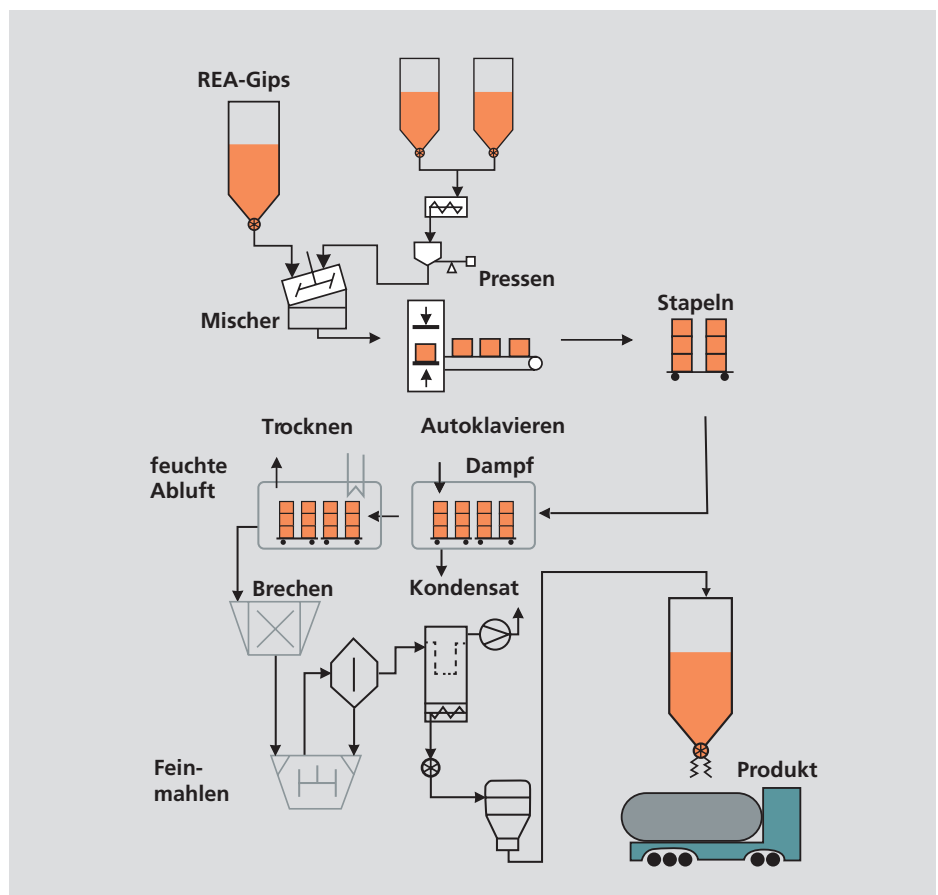
Abb. 8: Die Bildung von Calciumsulfat-Alpha-Halbhydrat aus REA-Gips
