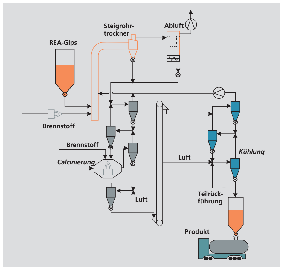
Abb. 11: Die Bildung von Thermischem Anhydrit aus REA-Gips
