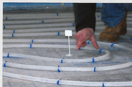
Messstelle im Heizstrich, wo die CM-Messung durchgeführt werden kann ohne eine Heizschlange zu beschädigen.
