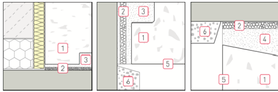
Abbildung 1: Konstruktionsdetails elastischer Anschlüsse an angrenzende Bauteile
